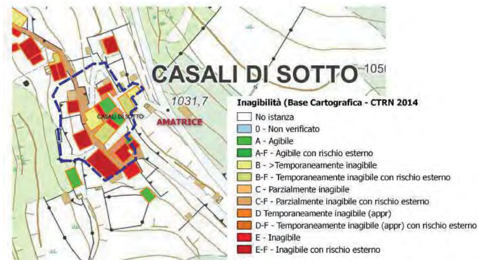
Figura 5 - Livello di Inagibilità degli edifici (schede AEDES) – Casali di Sotto
