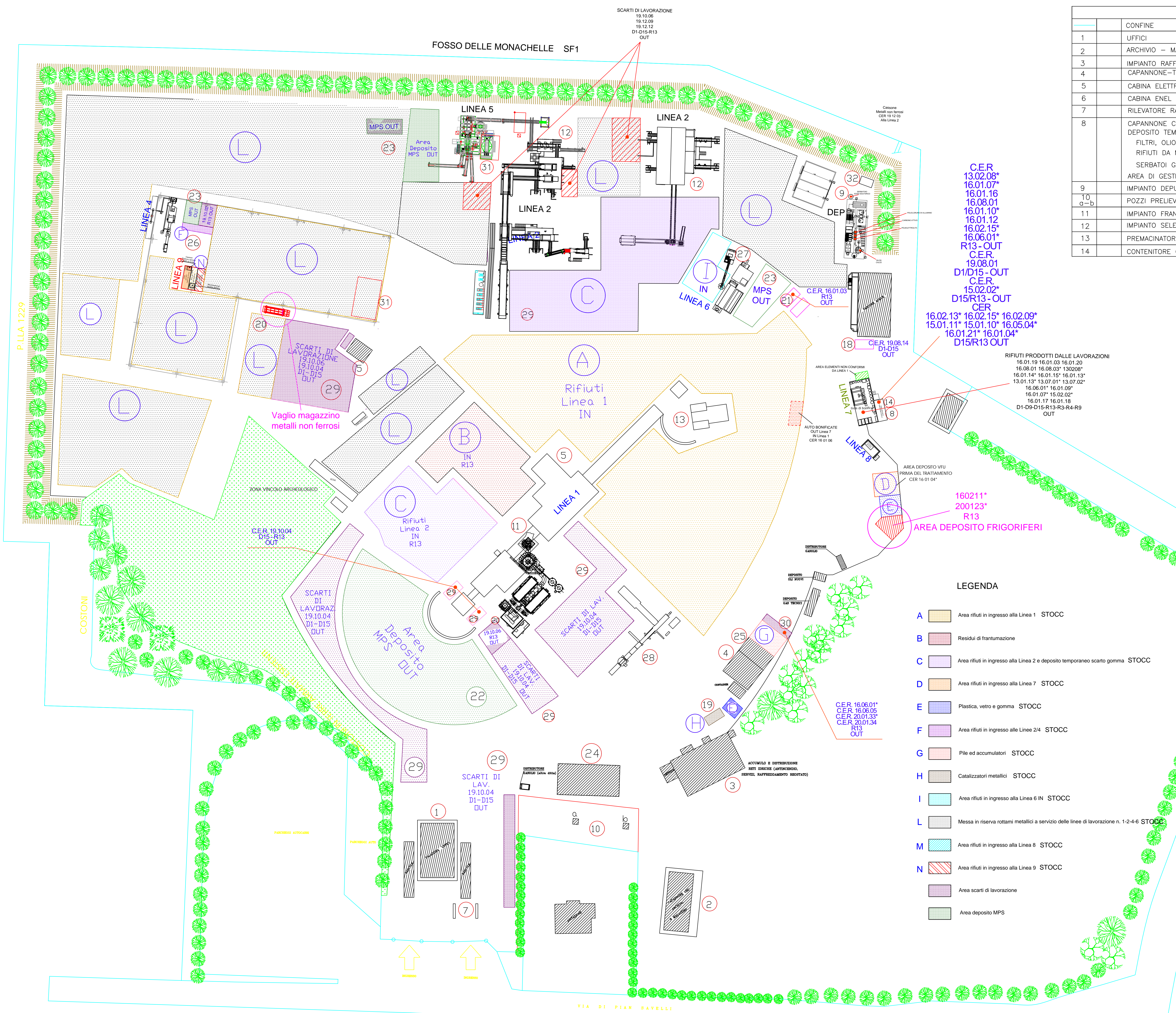
Planimetria generale delle aree scala 1:500
