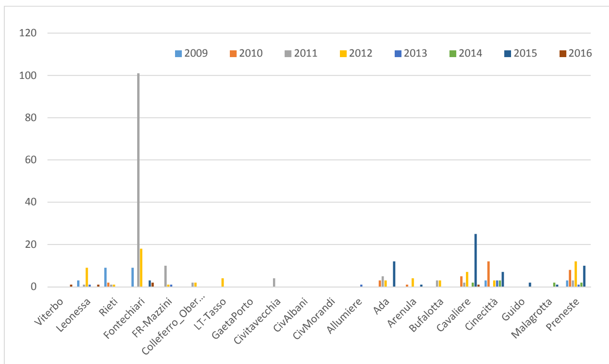
Figura 7.1 superamenti soglia informazione 180 µg/m 3
