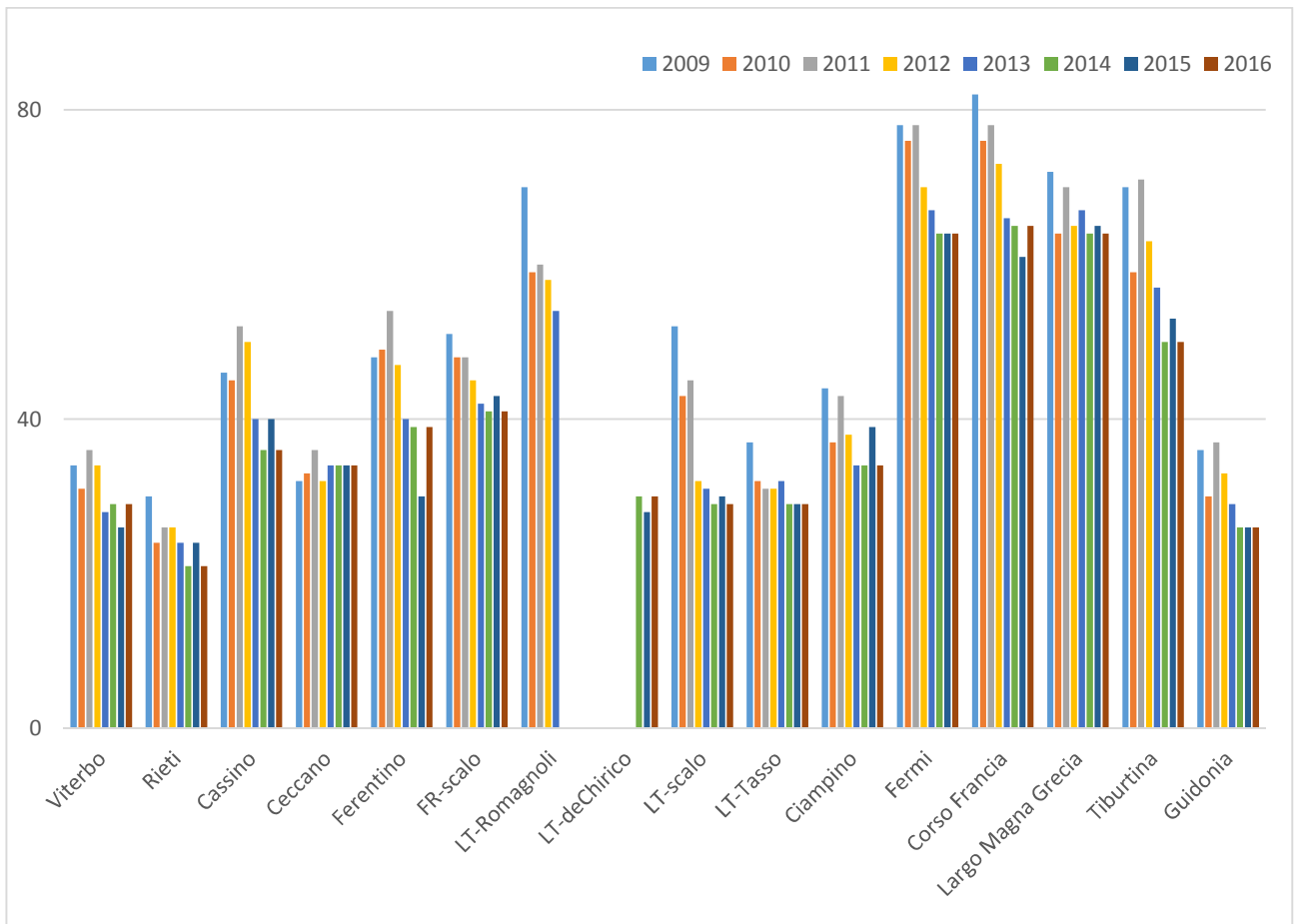
Figura 6.3 medie annue di NO 2 stazioni da traffico
