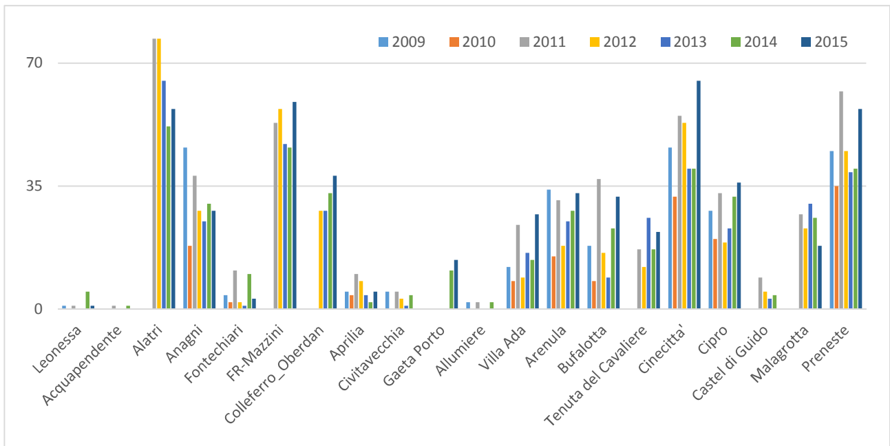
Figura 5.1.5 media giornaliera PM10 numero di superamenti dei 40 µg/m³ nelle stazioni di fondo
