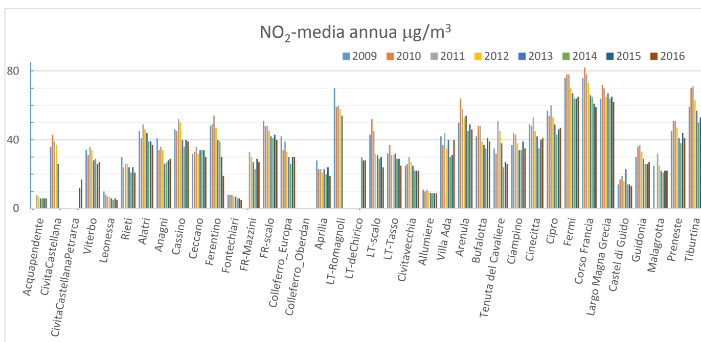
Figura 6.1 Medie annue di NO 2 2009-2016
