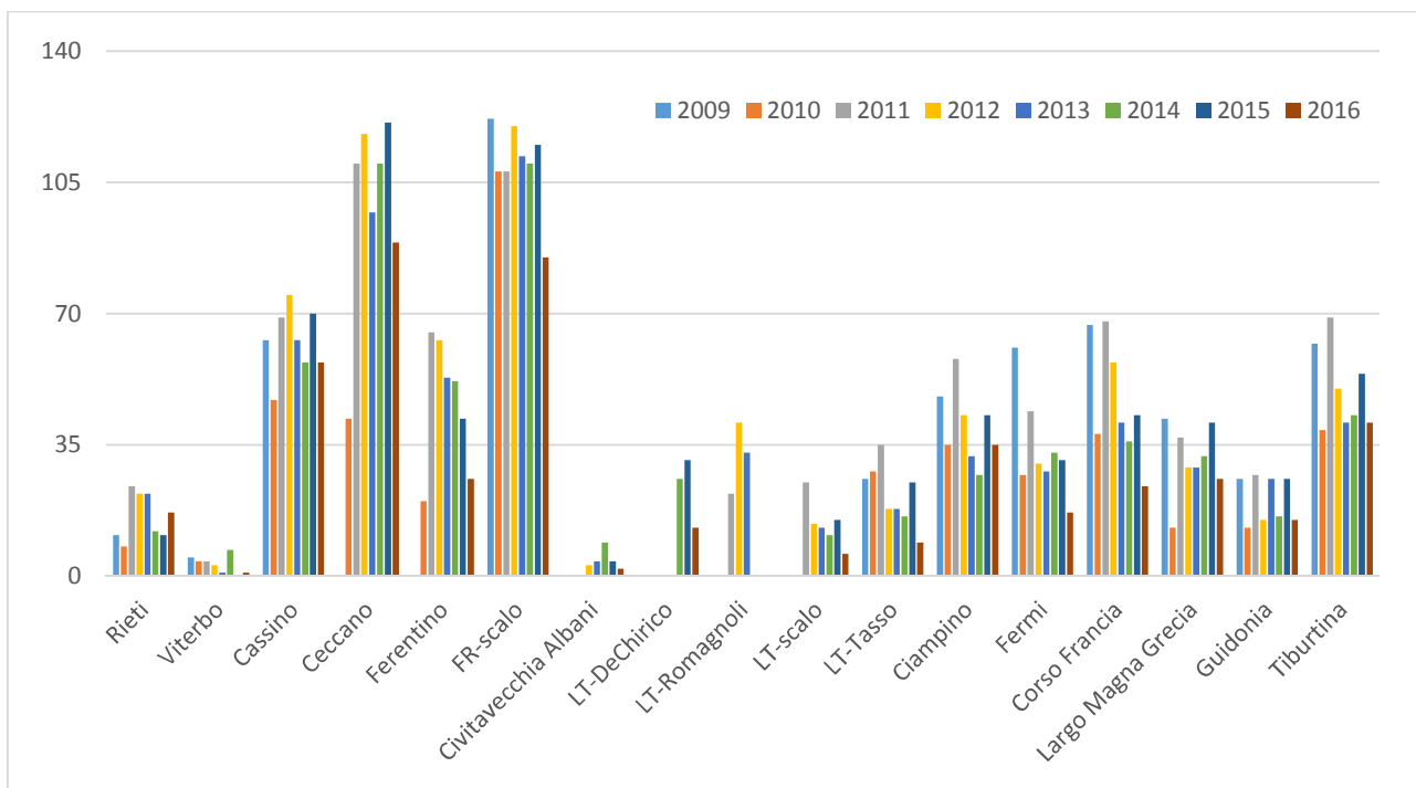
Figura 5.1.6 media giornaliera PM10 numero di superamenti dei 40 µg/m³ nelle stazioni da traffico
