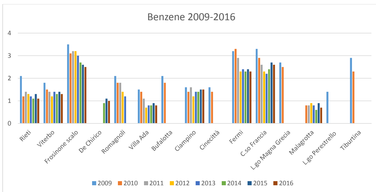
Figura 2.1 Media annua Benzene 2009-2016
