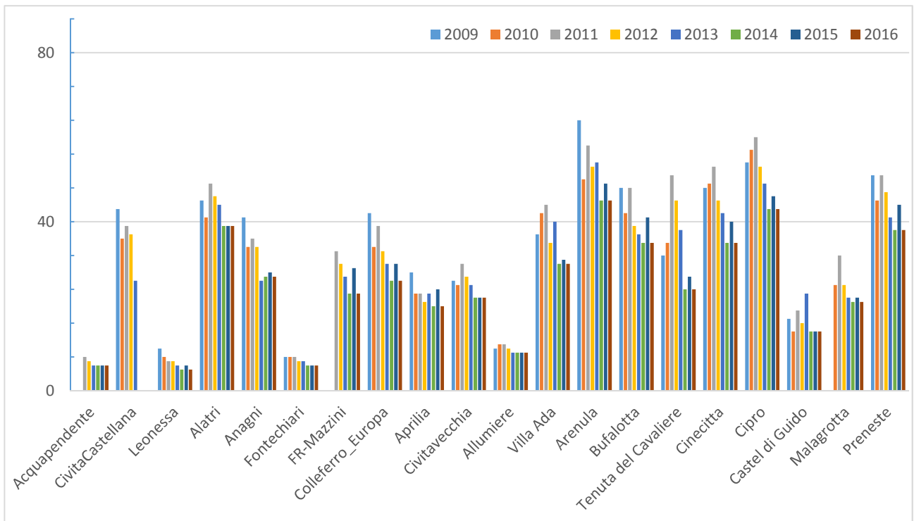
Figura 6.2 medie annue di NO 2 stazioni di fondo
