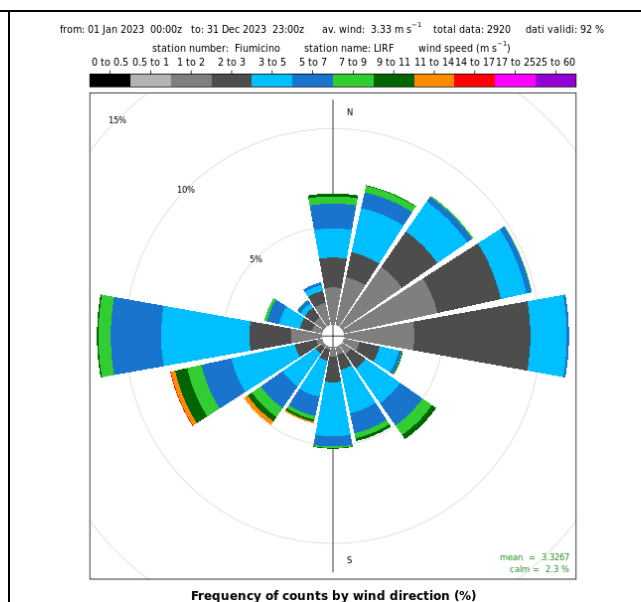
Figura 3.5 - Rosa dei venti di Fiumicino (16242 - LIRF) anno 2023.
