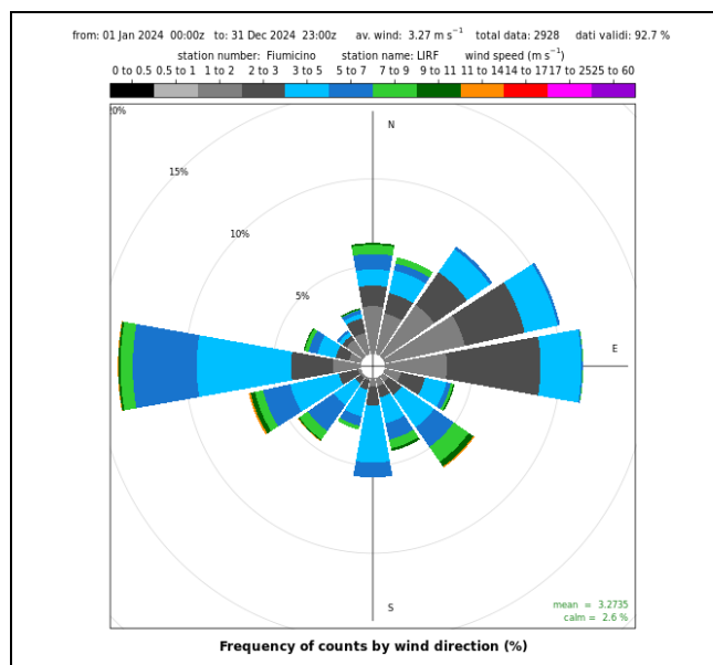
Figura 3.4 - Rosa dei venti di Fiumicino (16242 - LIRF) anno 2024.
