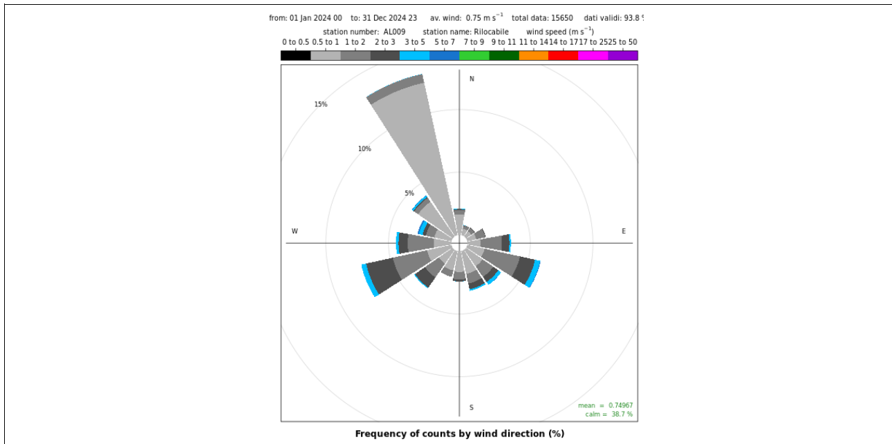
Figura 3.3 - Rose dei venti 2024 nelle stazioni della RMR.
