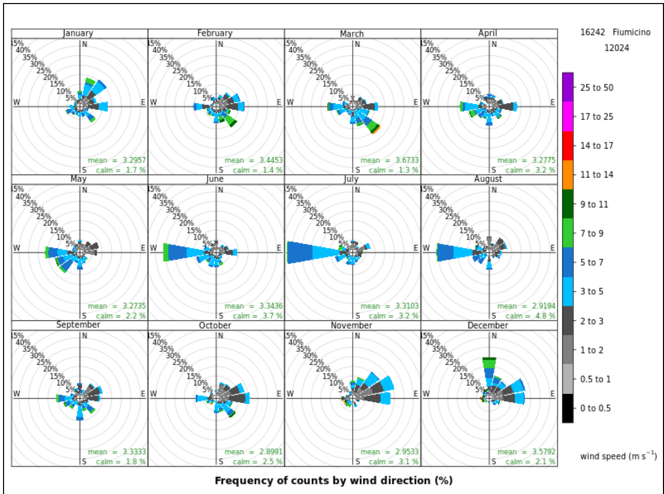
Figura 3.6 - Rosa dei venti di Fiumicino (16242 – LIRF) suddivisa per mese, anno 2024.
