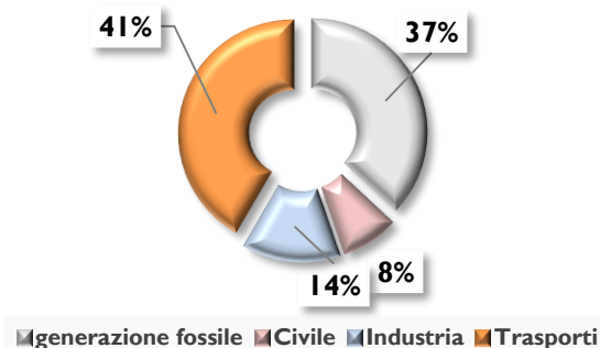
Emissioni CO 2 2050 - Lazio (Scenario Obiettivo)
