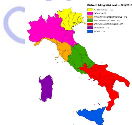
Figura 4: Distretti idrografici italiani definiti dalla L. 221/2015. Fonte: https://www.isprambiente.gov.it/pre_meteo/idro/UoM_CA.html
