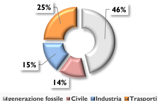
Emissioni CO 2 2030 - Lazio (Scenario Obiettivo)
