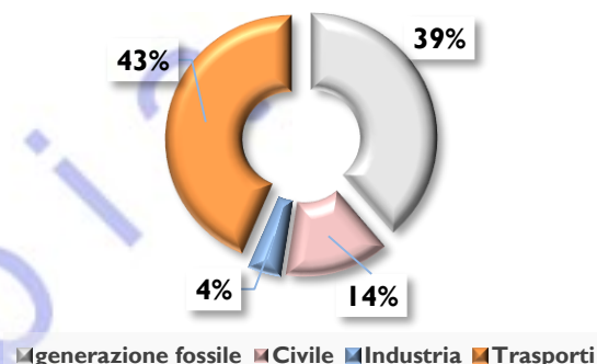
Emissioni CO 2 2050 - Lazio (Scenario Obiettivo)
