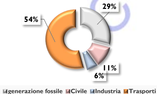
Emissioni CO 2 2030 - Lazio (Scenario Obiettivo)
