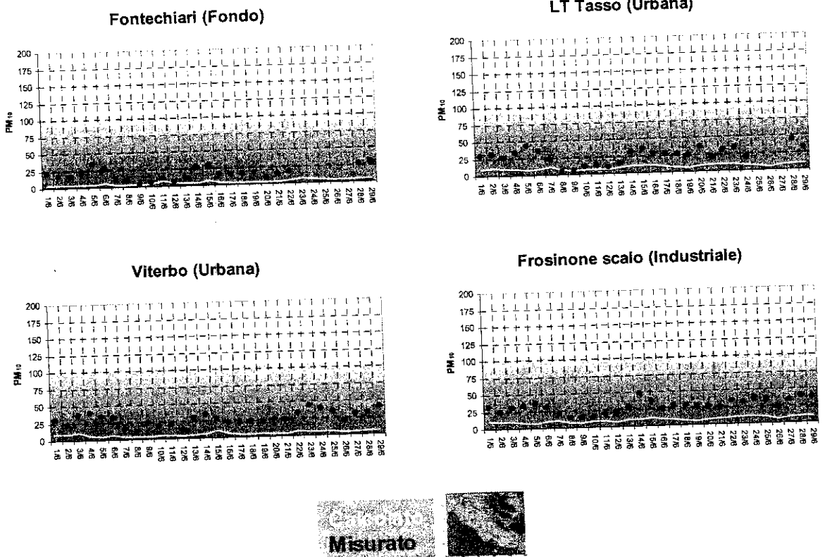
Figura 3.40 – Concentrazioni medie giornaliere osservate e calcolate di PM 10 [µg m -3 ] relativamente al mese di giugno 2005 (dominio regionale).
