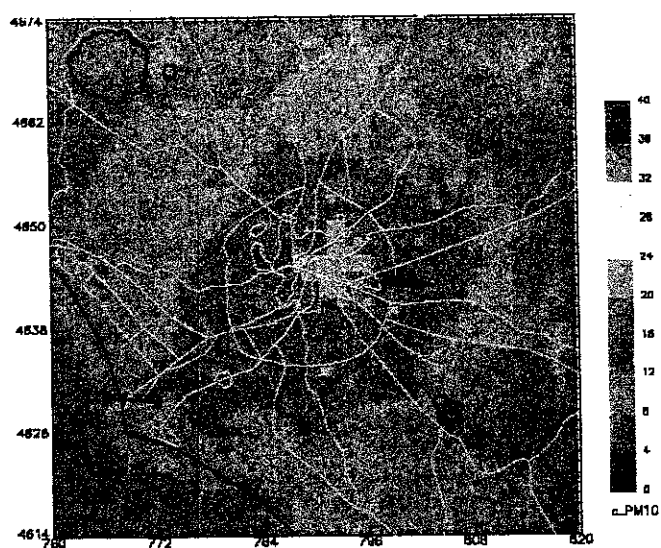
Figura 6.41 – Concentrazioni “medie annuali” di PM10 calcolate mediante l'utilizzo della (1).
