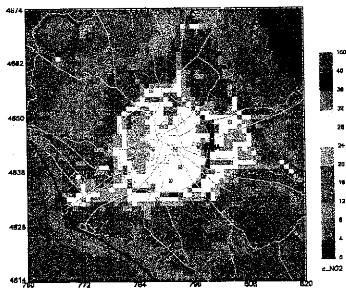
Figura 6.39 – Concentrazioni “medie annuali” di NO2 calcolate mediante l'utilizzo della (1).
