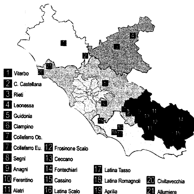
Figura 2.52 - Localizzazione delle stazioni di misura della rete di monitoraggio della qualità dell'aria al di fuori del comune di Roma
