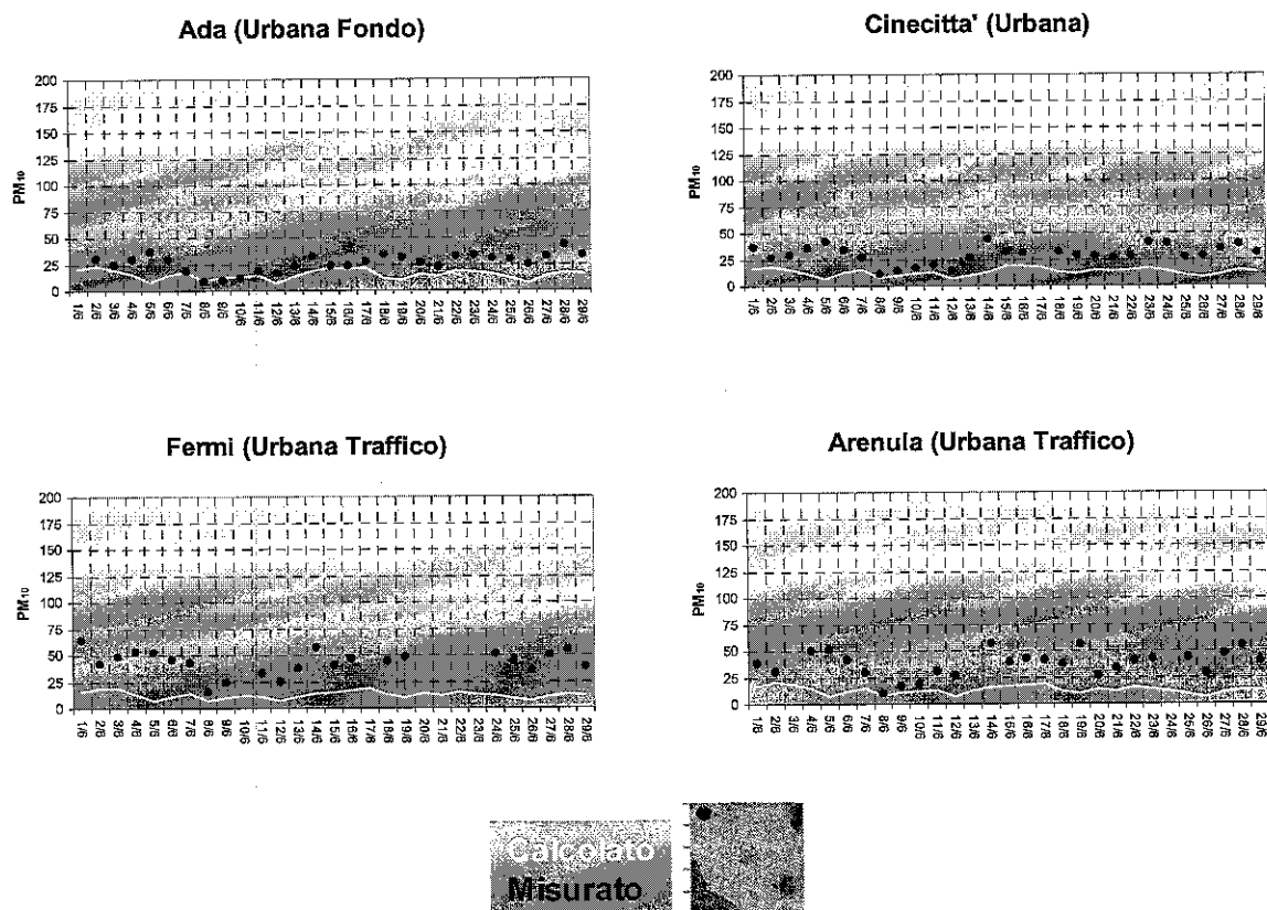
Figura 3.38 – Concentrazioni medie giornaliere osservate e calcolate di PM_{10} [ \mu g m^{-3} ] relativamente al mese di giugno 2005 (dominio locale).
