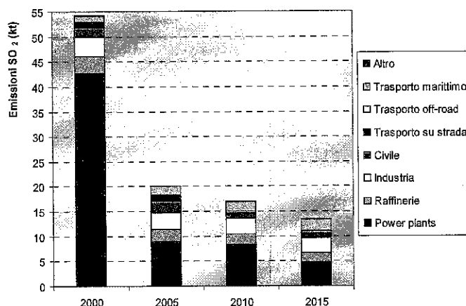
Emissioni SO2 - scenario CLE - LAZIO.
