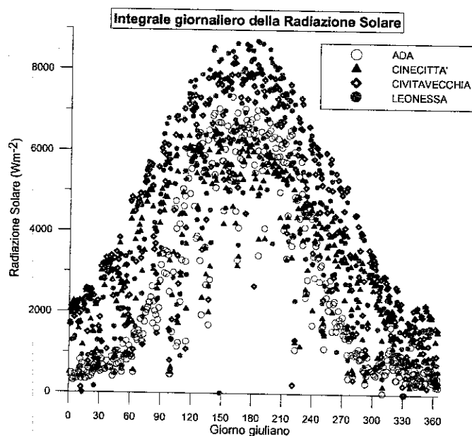
Figura 2.35 - Integrale giornaliero della radiazione solare rilevata al suolo nelle stazioni: Ada, Cinecittà, Civitavecchia e Leonessa nel 2005.
