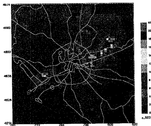
Figura 6.45 – Concentrazioni “medie annuali” di SO2 calcolate mediante l'utilizzo della (1).
