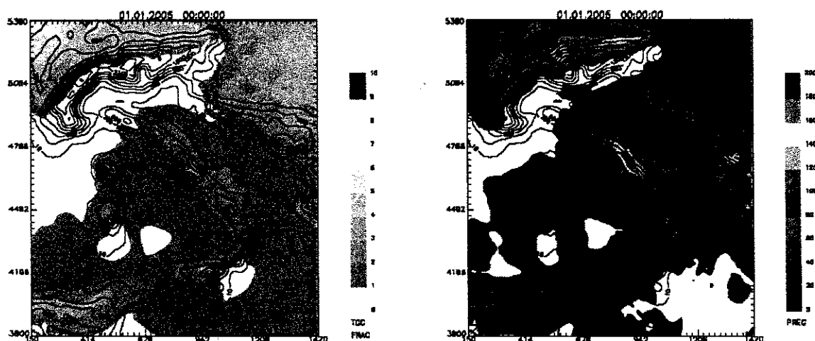
Figura 3.7 - Valori medi mensili di copertura nuvolosa (sinistra) e precipitazione cumulata (destra), per il mese di gennaio 2005
