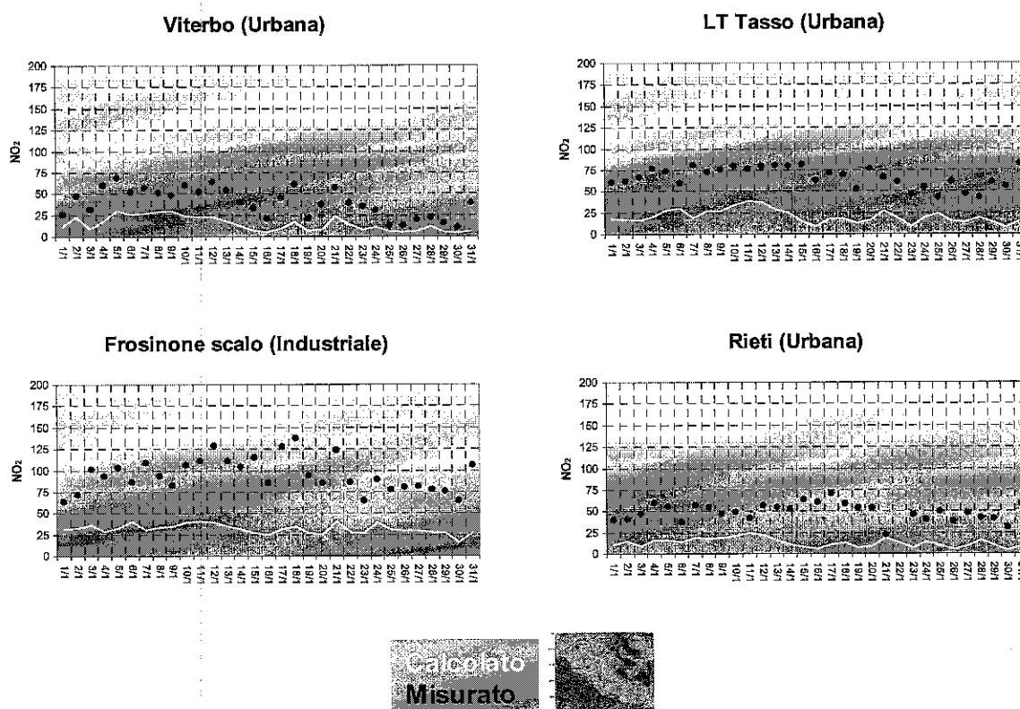
Figura 3.36 – Concentrazioni medie giornaliere osservate e calcolate di \text{NO}_2 [ \mu\text{g m}^{-3} ] relativamente al mese di gennaio 2005 (dominio regionale).
