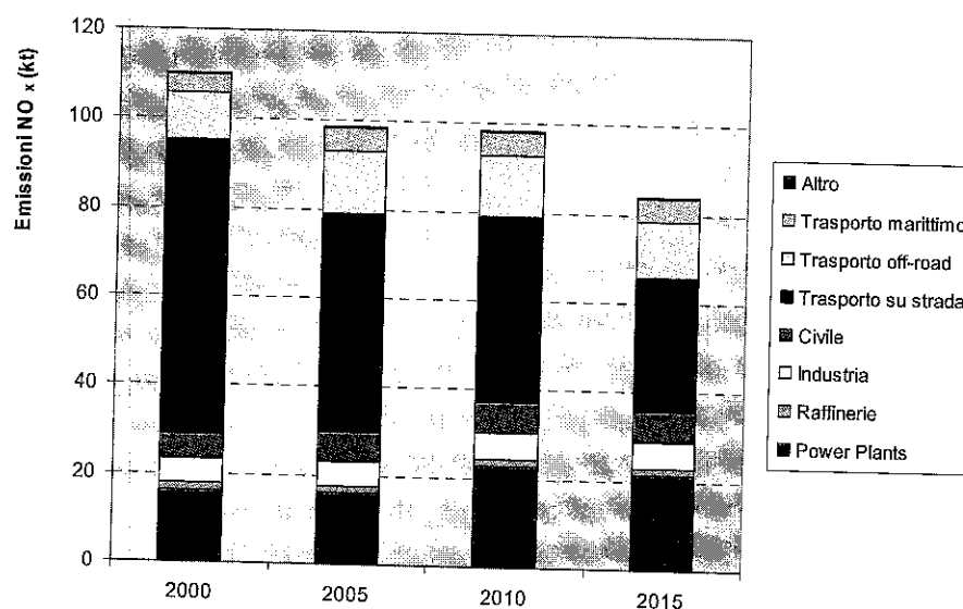
Figura 6.2 – Emissioni NO x - scenario CLE - LAZIO.
