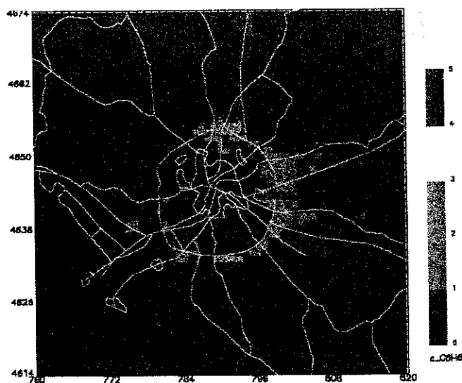
Figura 6.43 – Concentrazioni “medie annuali” di C6H6 calcolate mediante l'utilizzo della (1).
