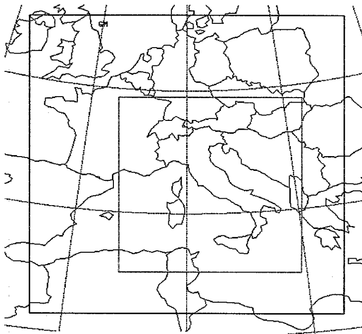
Figura 3.4 - Domini di calcolo esterno (risoluzione 60x60 km 2 ) e nazionale (risoluzione 20x20 km 2 ) del modello MINNI.
