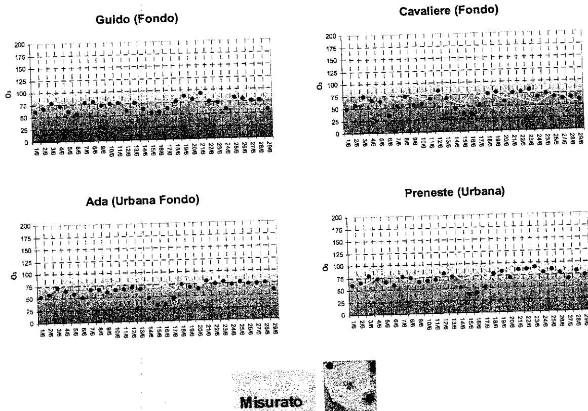
Figura 3.41 – Concentrazioni medie giornaliere osservate e calcolate di O 3 [µg m -3 ] relativamente al mese di giugno 2005 (dominio locale).
