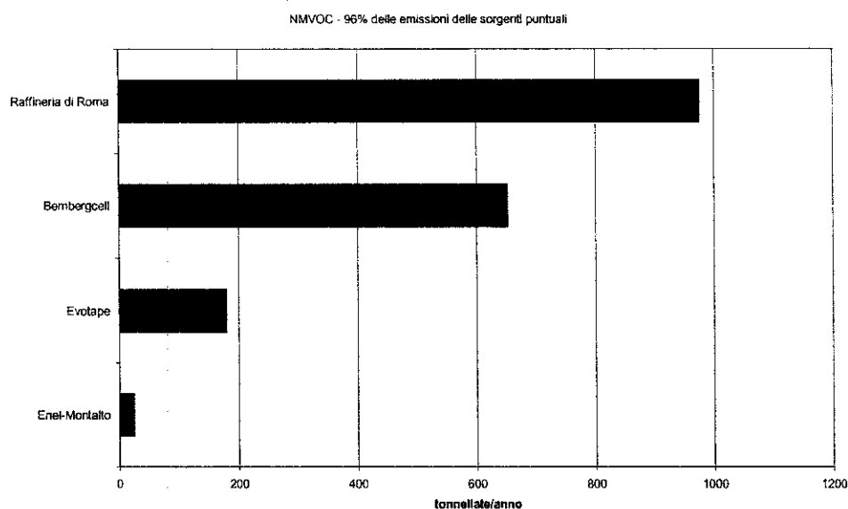
Figura 2.19 –Emissioni di NMVOC rappresentative del 96% del totale.
