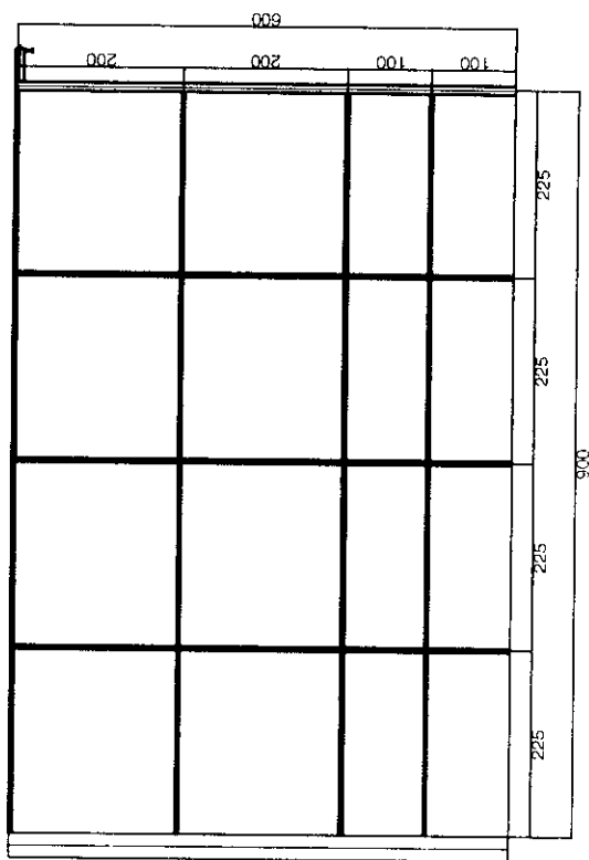
Elemento divisorio (rastrelliera) scala 1:100
