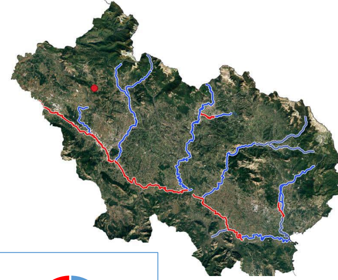
STATO CHIMICO 2021-2023
