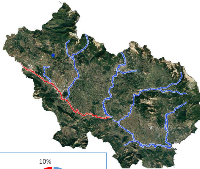
STATO CHIMICO 2018-2020
