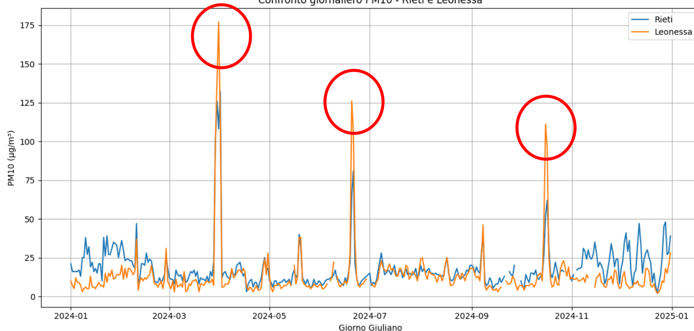
Confronto giornaliero PM10 - Rieti e Leonessa
